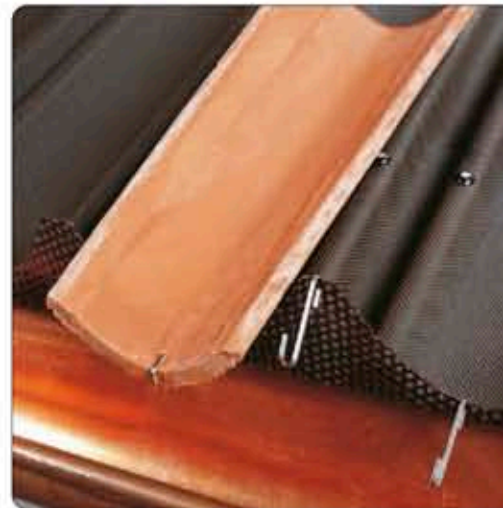
3. lépés: helyezze a rácshoz tartozó induló cseréprögzítő kampókat az erre a célra szolgáló lyukakba, és akassza be a kolostor cserepeket.
