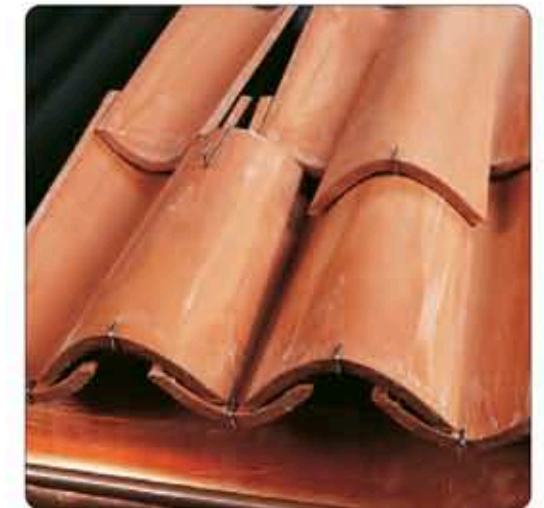
5. lépés: folytassa a tetőfedést, helyezze el a kolostorcserépekhez való felsőcserep rögzítő kampókat (négyzetméterenként kb. 15 db).
