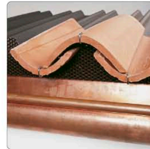
4. lépés: a beakasztott cserepek és a rácshoz tartozó részlete, amely lehetővé teszi a tető szellőzését.
