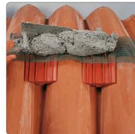
8. lépés: vigye fel a habarcst a háló hosszában a nyílás fölé.
