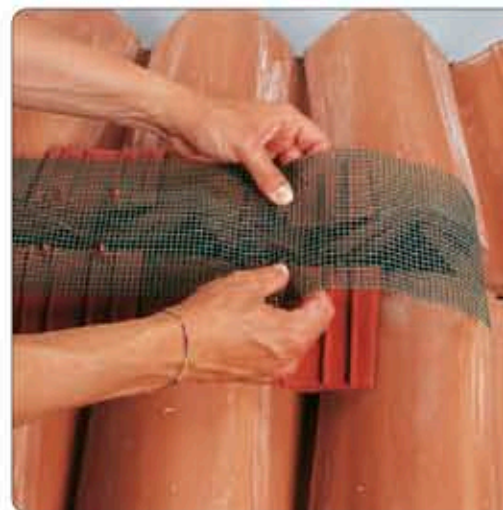
7. lépés: nyomja rá a zöld habarcstartó műanyag hálót a nyílások támaszaira.
