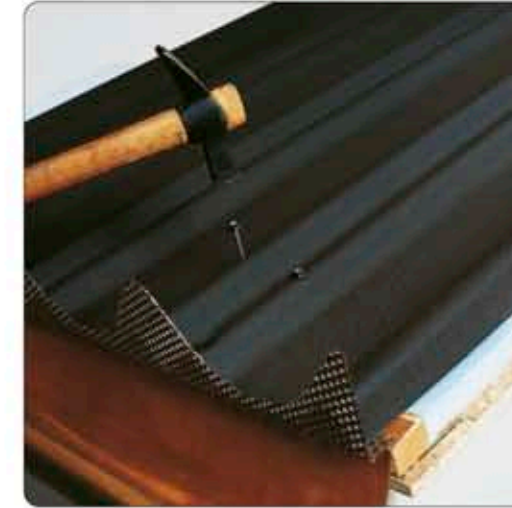
2a. lépés: helyezze el a gutta bitumenes lemezt, és rögzítse a faszervezethez gutta szögekkel...
